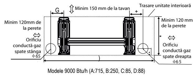
Modele 9000 Btu/h (A:715, B:250, C:85, D:88)
