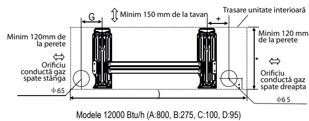
Modele 12000 Btu/h (A:800, B:275, C:100, D:95)
