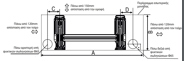
Μοντέλα 12.000Btu/h(A:800, B:275, C:100, D:95)
