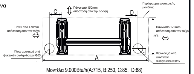
Μοντέλα 9.000Btu/h(A:715, B:250, C:85, D:88)
