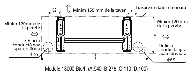
Modele 18000 Btu/h (A:940, B:275, C:110, D:100)
