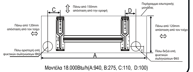
Μοντέλα 18.000Btu/h(A:940, B:275, C:110, D:100)
